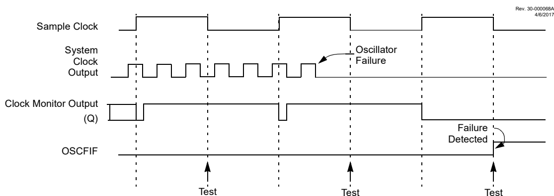
图 7-10. FSCM 时序图
