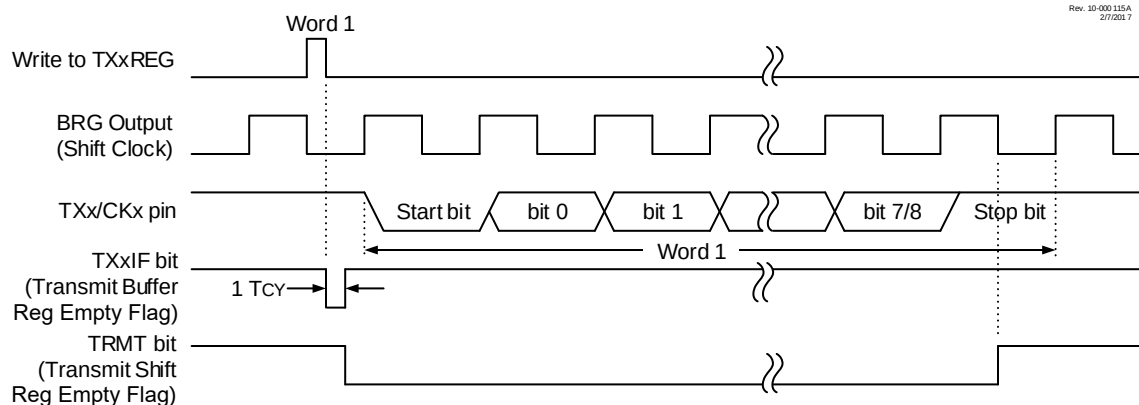
图 31-10. 同步发送
