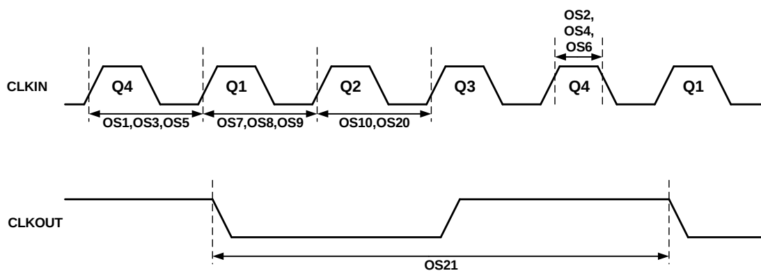
图 42-4. 时钟时序
