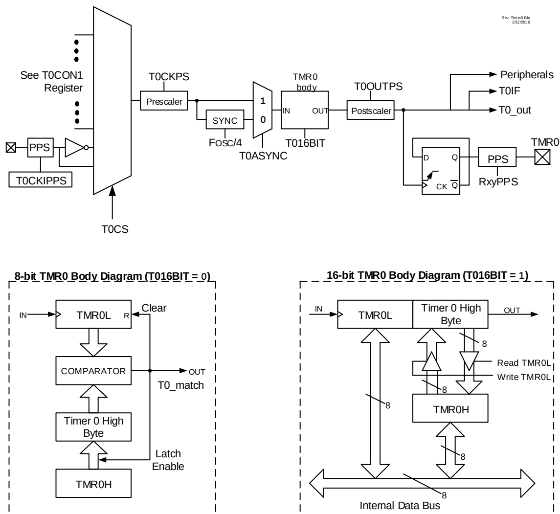
图 21-1. Timer0 框图
