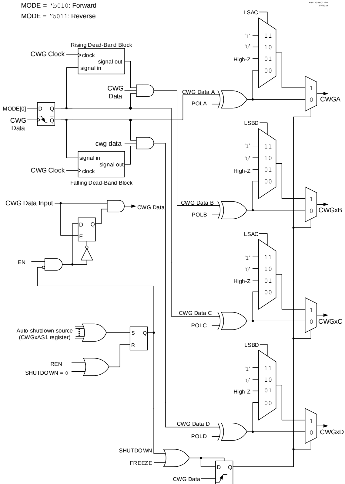
图 27-6. CWG 简化框图（正向和反向全桥模式）
