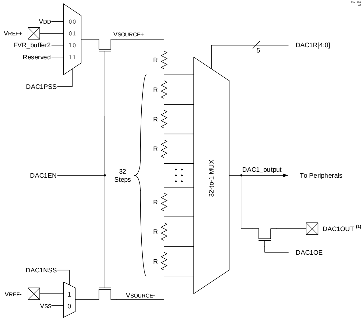
图 35-1. 数模转换器框图
