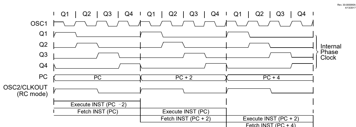
图 13-2. 时钟/指令周期
