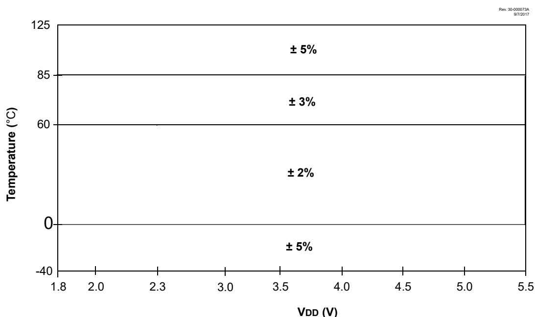
图 42-5. 器件 V_{DD} 和温度范围内的 HFINTOSC 频率精度（已校准）
