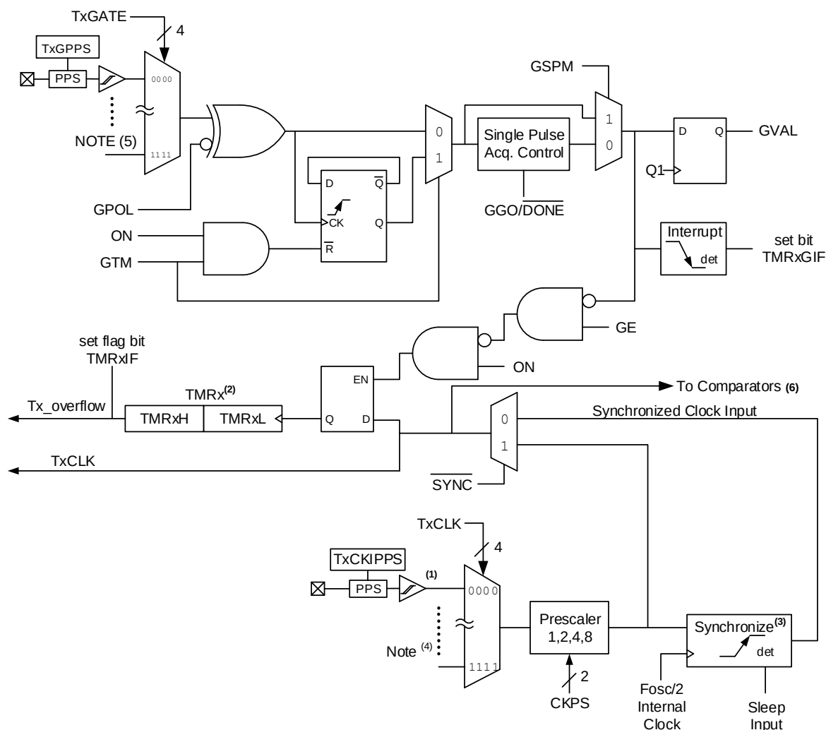
图 22-1. Timer1 框图
