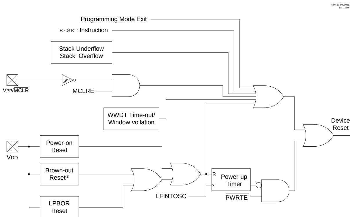
图 11-1. 片上复位电路的简化框图
