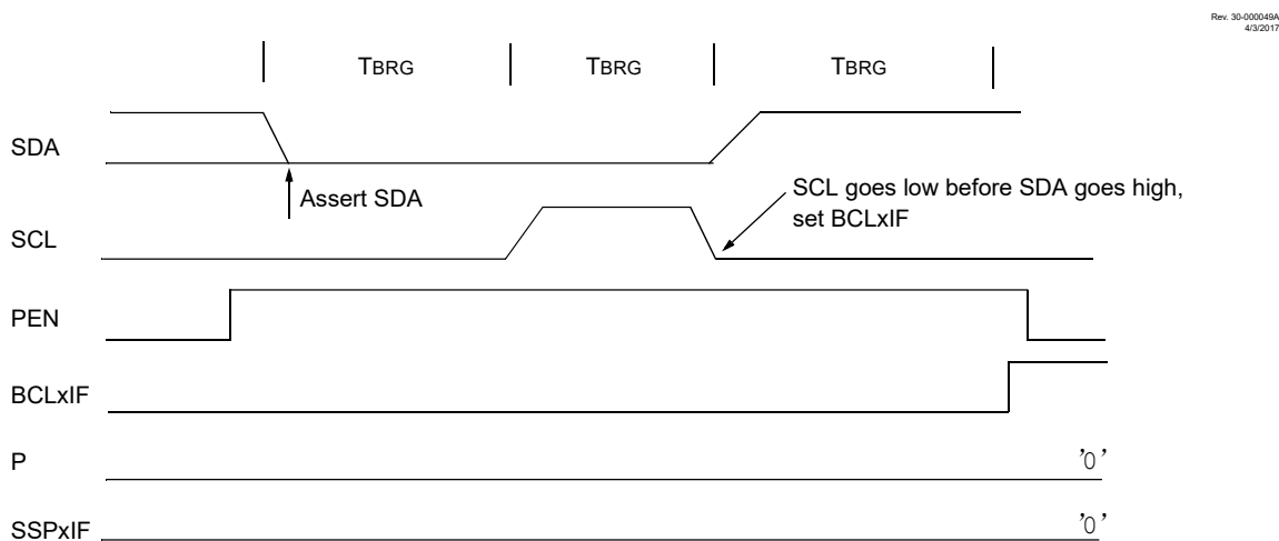
图 30-40. 停止条件期间的总线冲突（情形 2）
