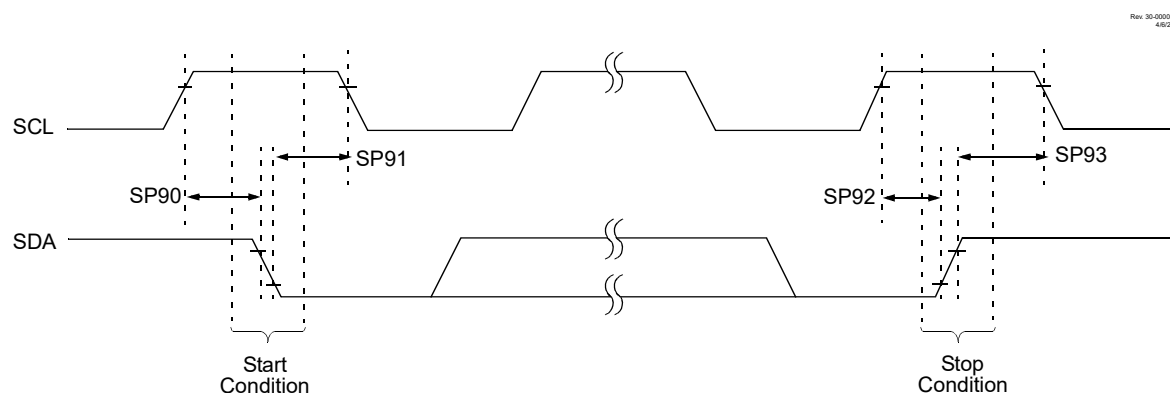
图 42-19. I 2 C 总线启动/停止位时序
