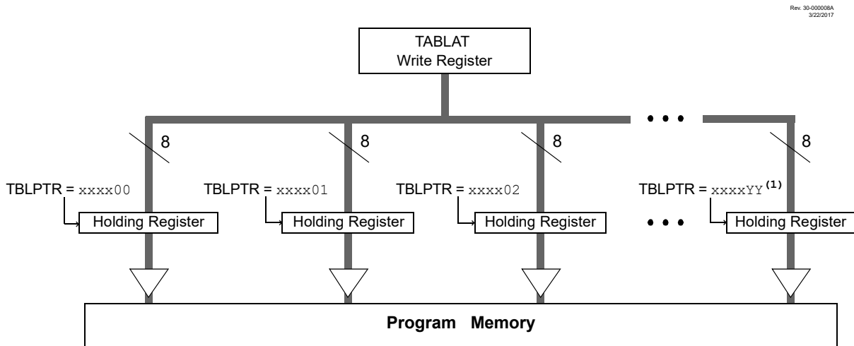
图 14-8. 对程序闪存进行表写
