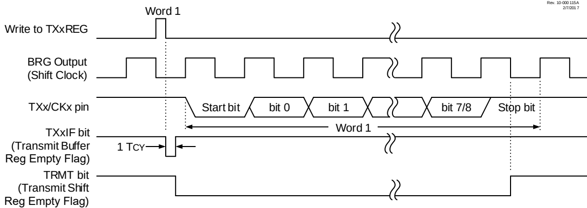
图 31-3. 异步发送
