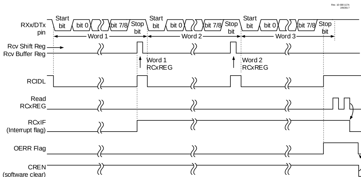
图 31-5. 异步接收
