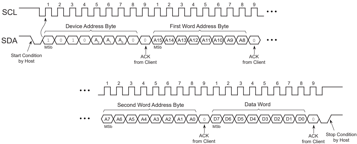
图 7-1. 字节写操作
