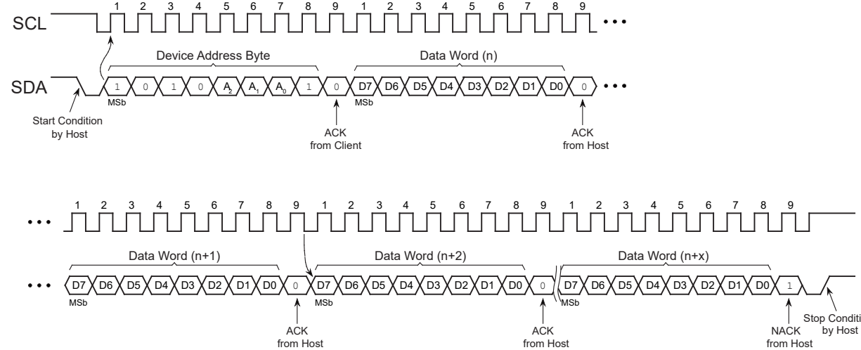
图 8-3. 连续读操作
