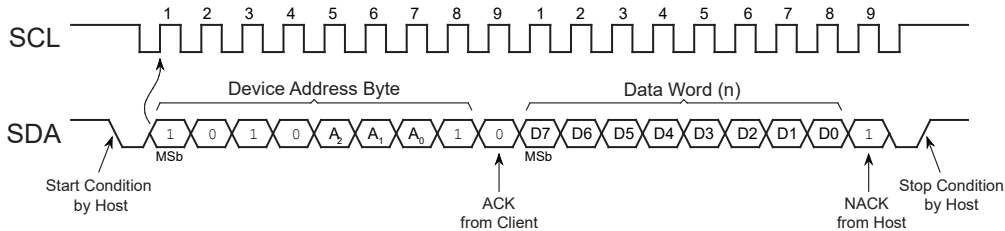
图 8-1. 当前地址读操作
