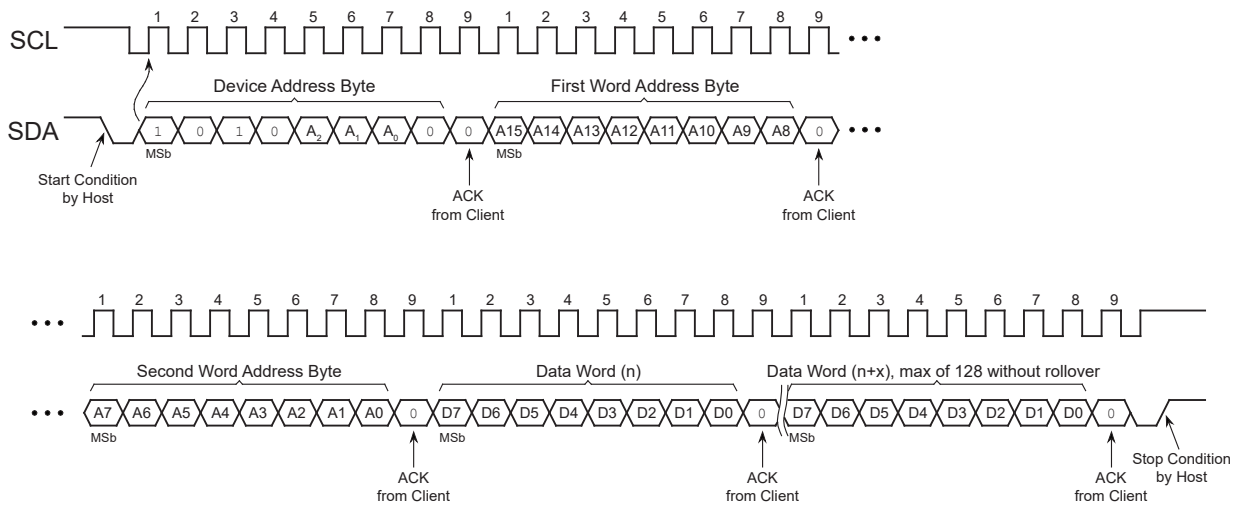
图 7-2. 页写操作
