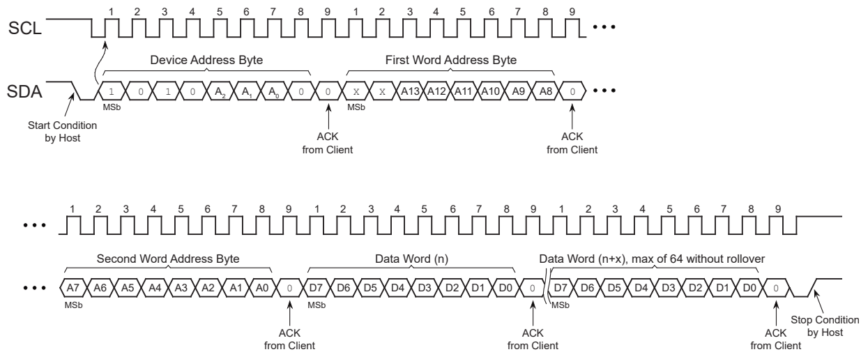
图 7-2. 页写操作
