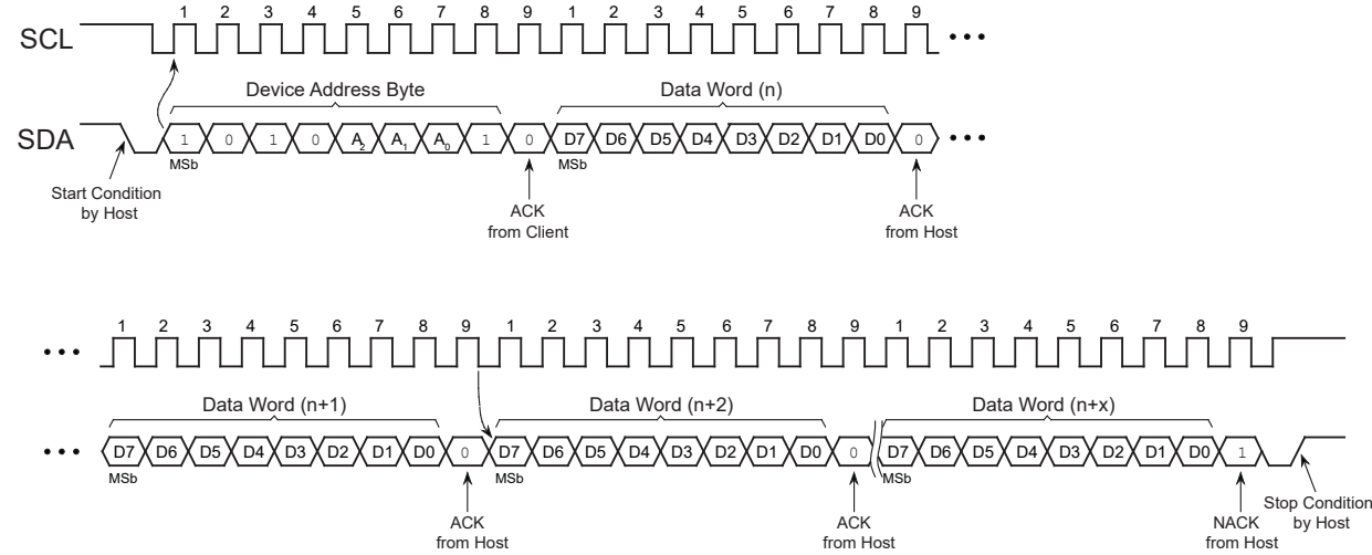
图 8-3. 连续读操作
