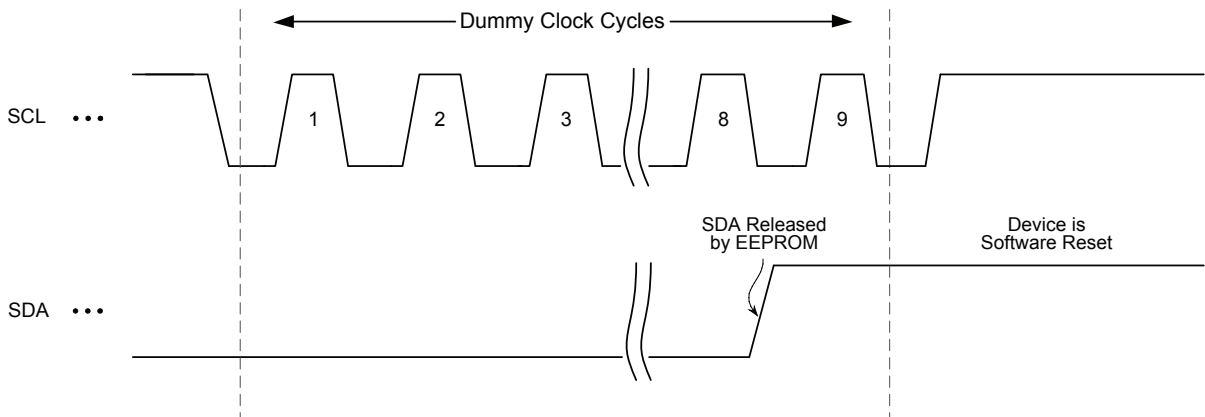
图 5-2. 软件复位
