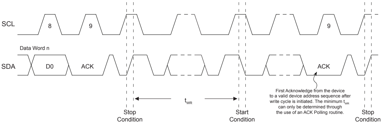
图 7-4. 写周期时序
