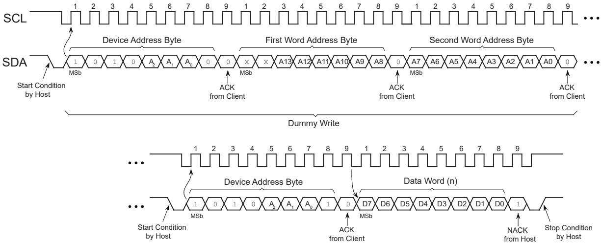
图 8-2. 随机读操作
