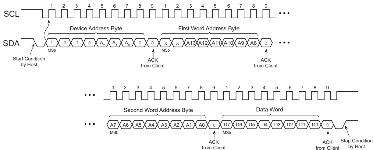
图 7-1. 字节写操作
